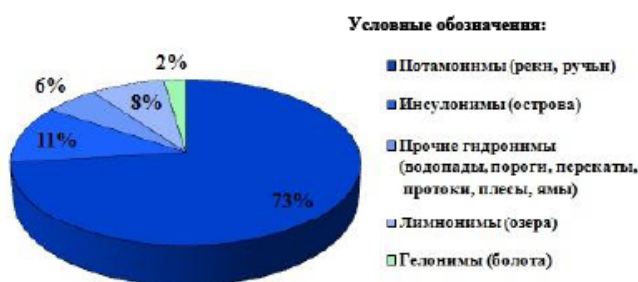
Рис. 6. Дифференциация гидронимии на основе отношения их к типу географического объекта. Fig. 6. Differentiation of hydronymy based on their relation to the type of geographical object.
