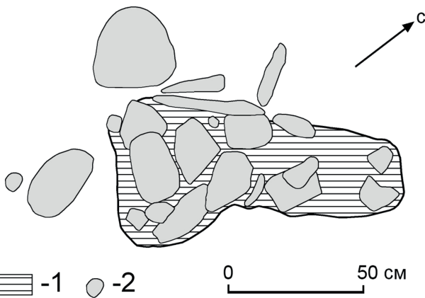
Рис. 5. Горн из каменных плит для производства железа на стоянке Пески IVa. 1 – углистый слой со шлаками; 2 – каменные плиты из уплощенных или расколотых валунов.
