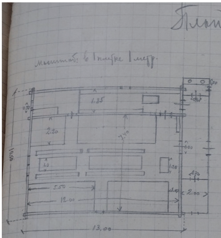
Рисунок 1. Рисунок типового барака для рабочих на лесозаготовках. Фрагмент 1. Источник. [14, Л. 28–29]. Pic. 1. Drawing of the typical barrack for logging workers. Fragment 1. Source. [14, Л. 28–29].
